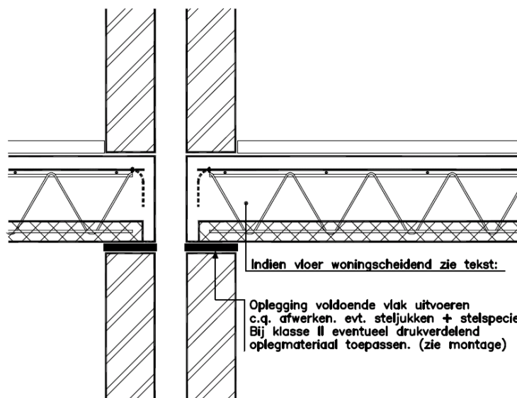
Detail 1a
