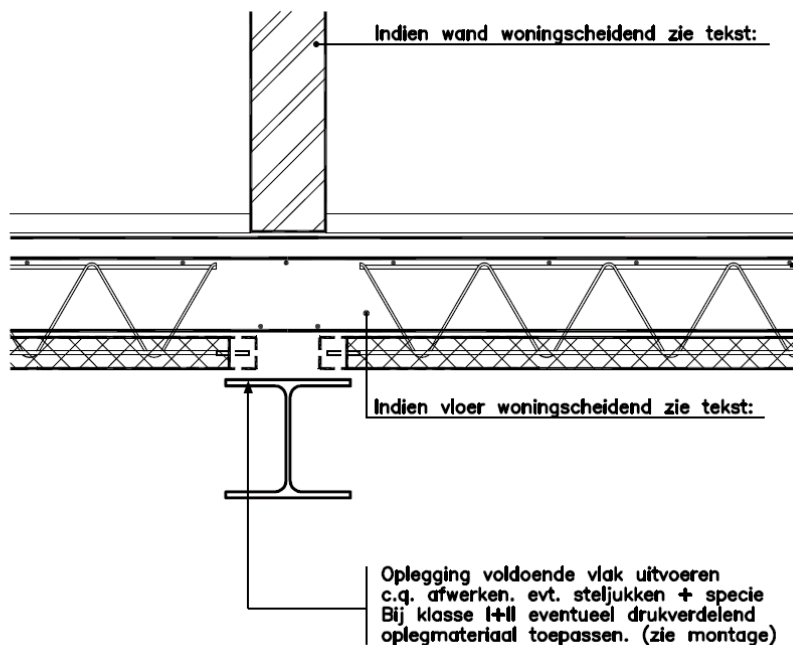
Detail Xa
